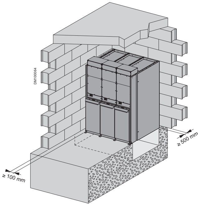
底部泄压内燃弧开关柜的布置
